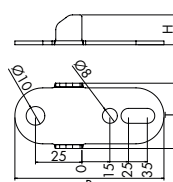
Wandbestimmungshalter Flach
